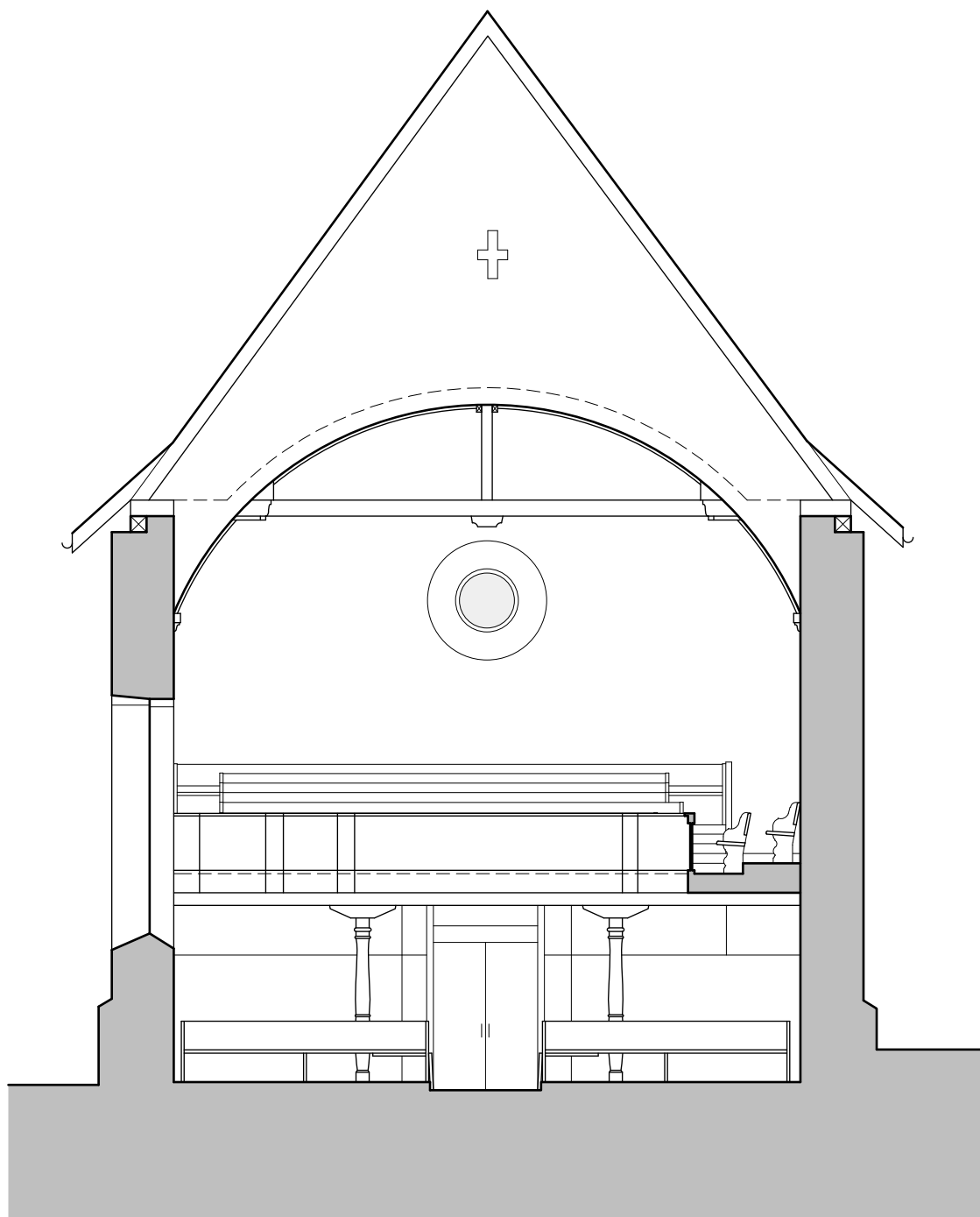
Ansicht Rückwand Schiff 1:100
