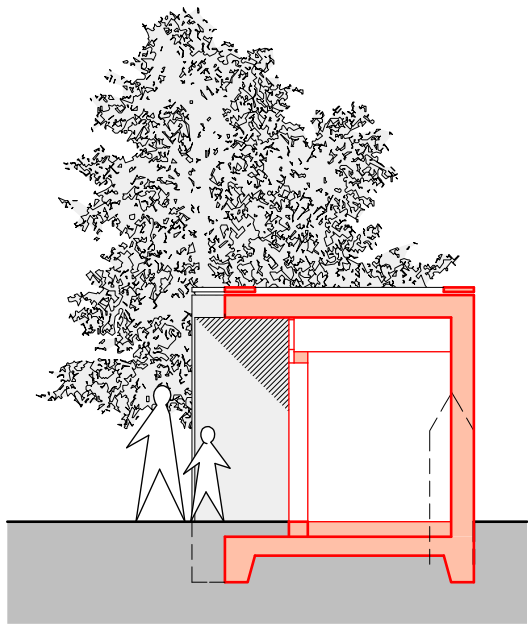
SCHNITT A
