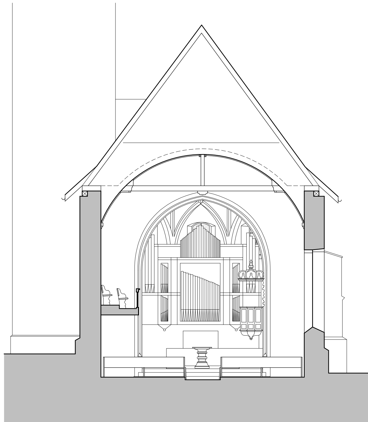
Ansicht Chorbogen 1:100
