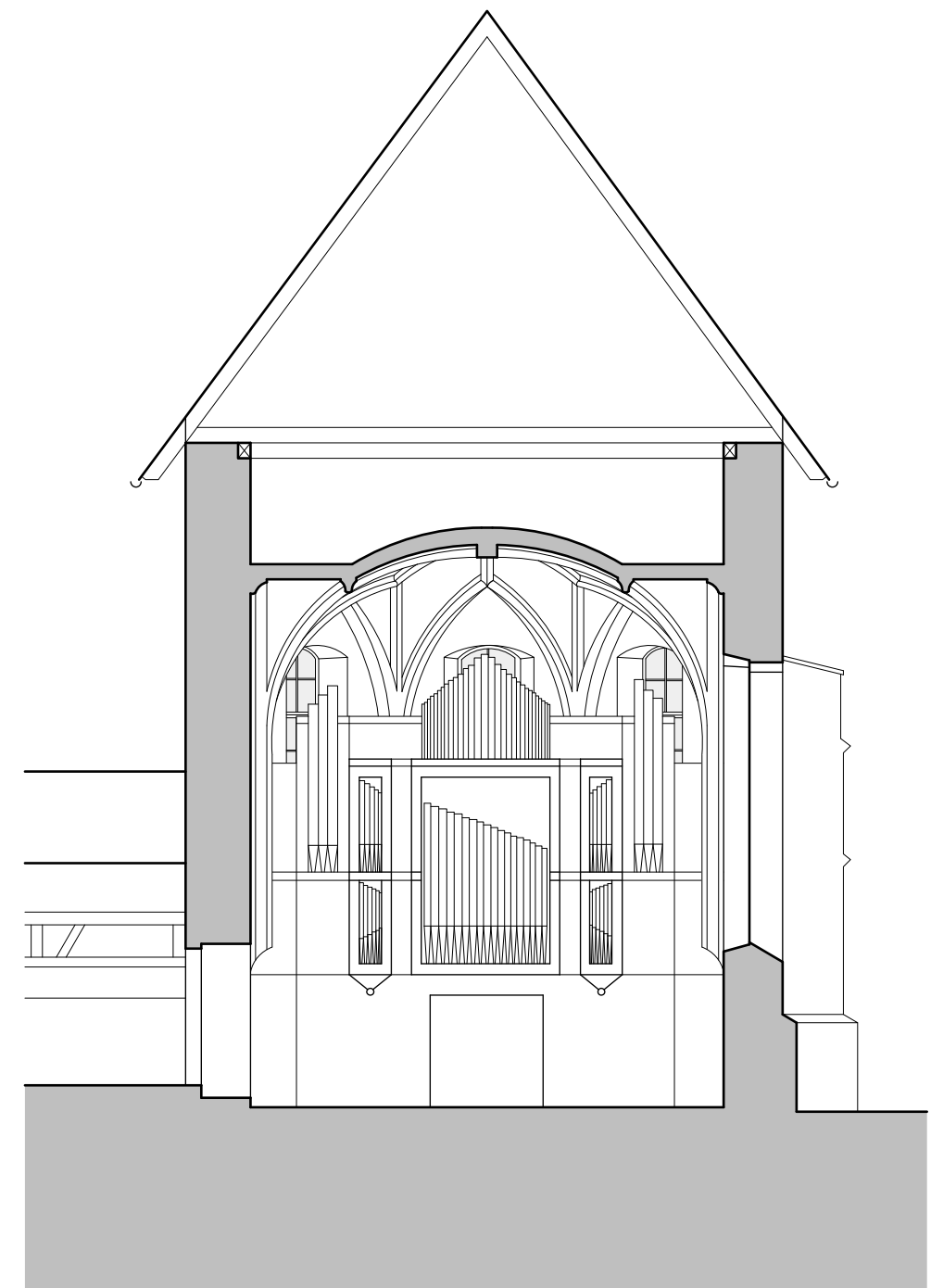
Querschnitt Chor bestehend 1:100
