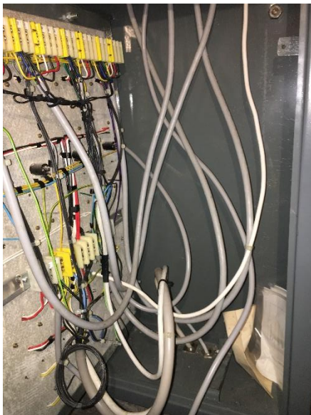
Verdrahtung im Tableau mit Kabel die abgetrennte Drähte in nicht isoliertem Zustand enthalten
